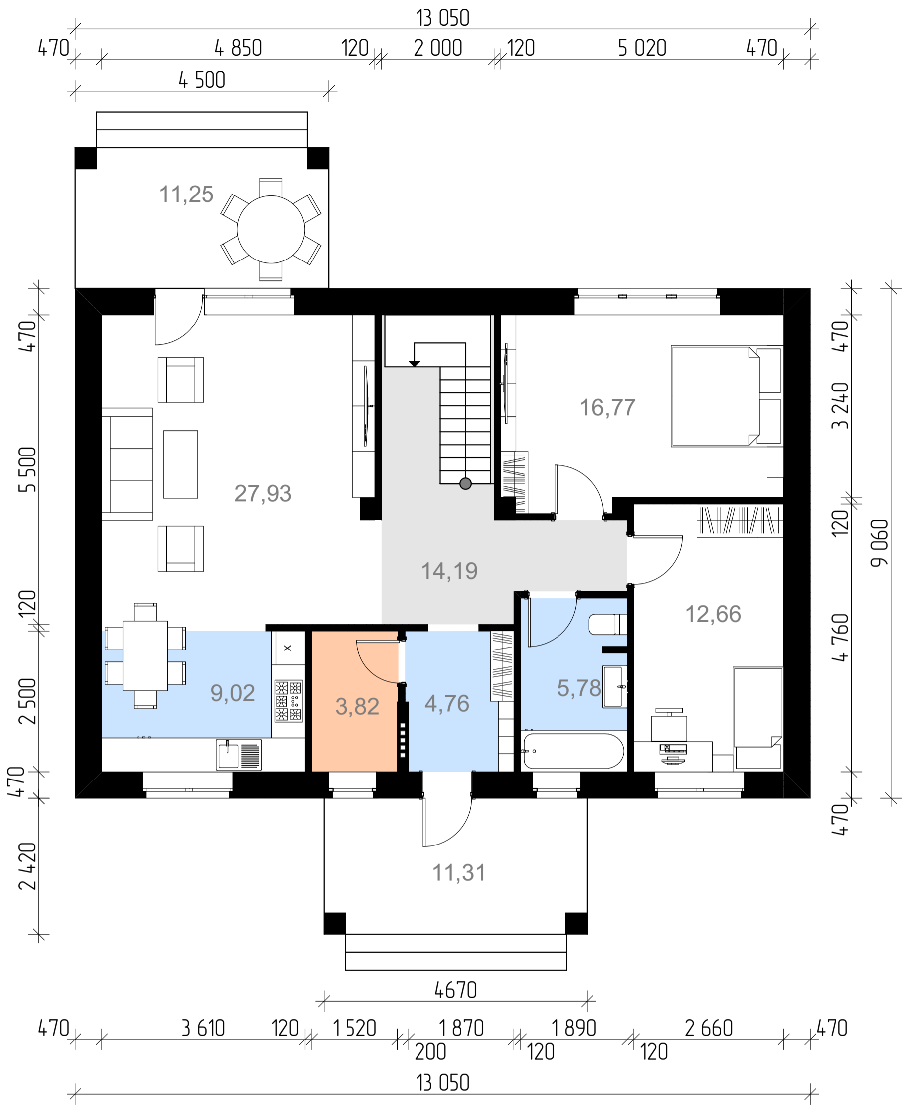
Экспликация 1 этажа
